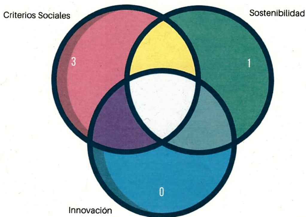
Gráfico 1. Diagrama de VENN de la incorporación de criterios de la CPISSR.
